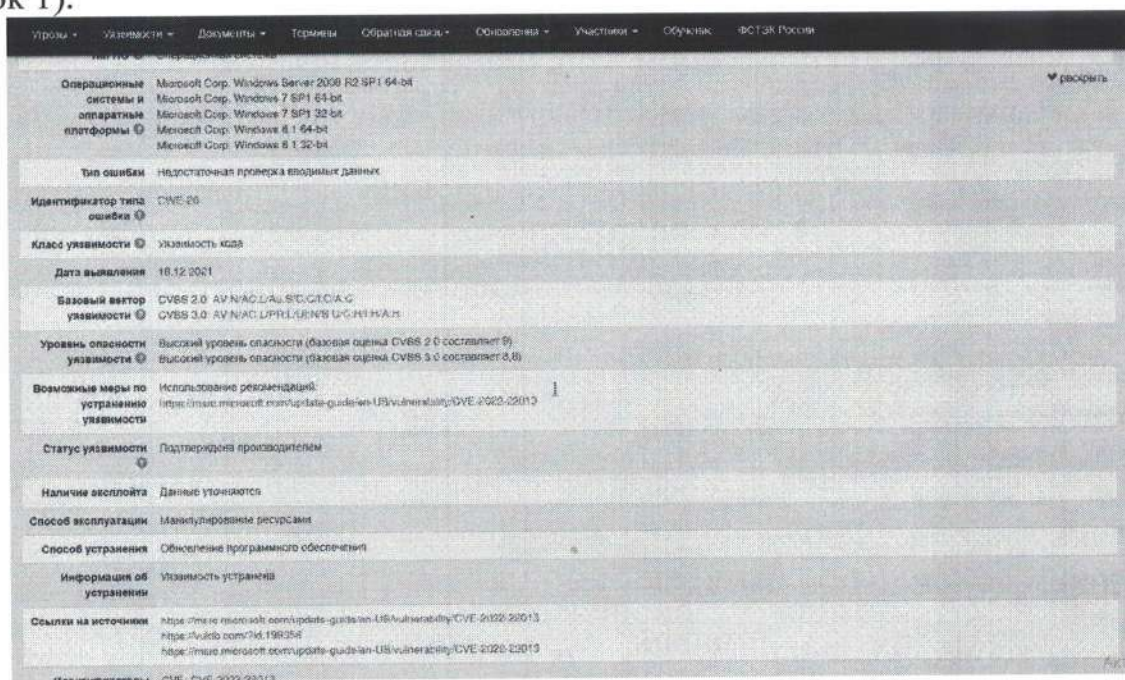
Рисунок 1. Расположение рекомендаций по устранению уязвимостей.
